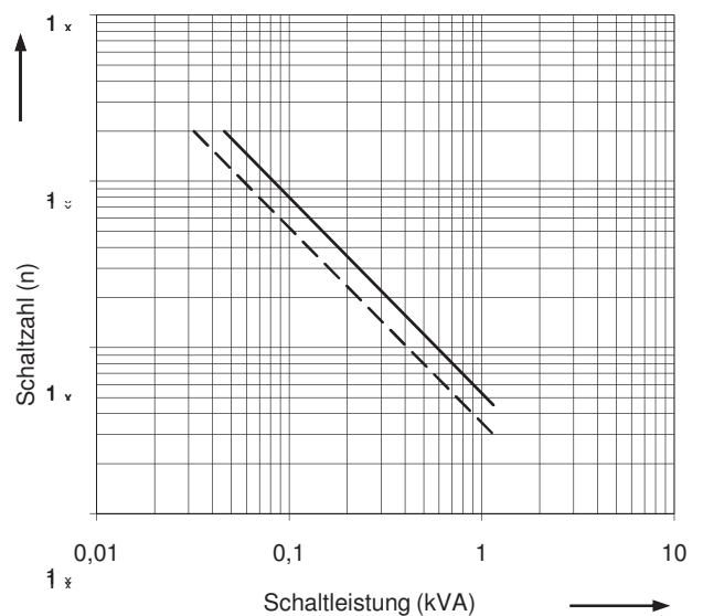
2 RH 02, 2RH 32, 2 RH 62, 4 RH 12, 4 RH 42 Kontaktwerkstoff AgCu
