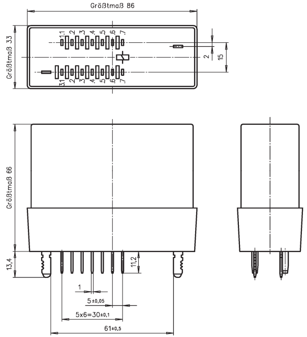
Maßbild Rs 805 495
