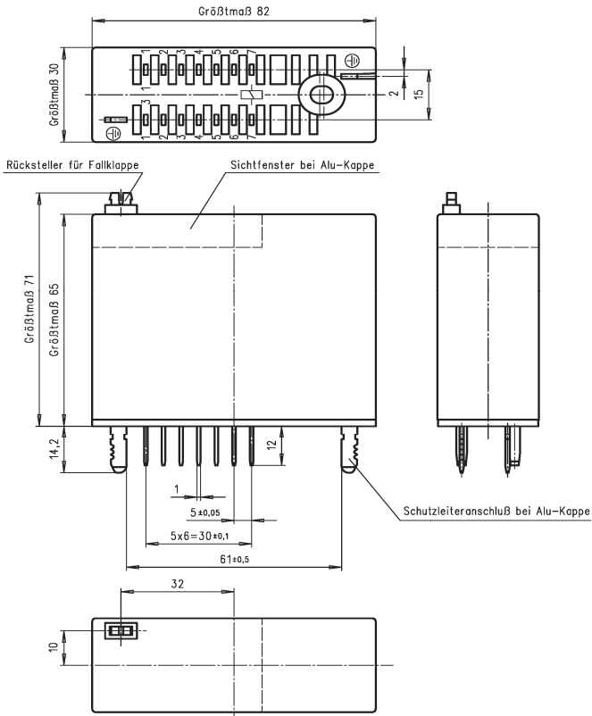
Maßbild Rs 805 540
