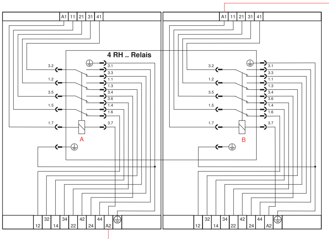
Verdrahtungsplan für RELOG - Schaltrelais 4 RH 10 / 4 RH 12 mit 2 Stück RELOG - Steckfassungen für SSB (DIN Kennzeichnung, ohne Freilaufdiode)
