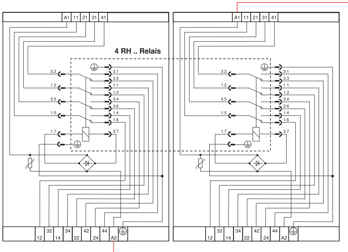
Verdrahtungsplan für RELOG - Schaltrelais 4 RH 40 / 4 RH 42 mit 2 Stück RELOG - Steckfassungen für SSB mit Brückengleichrichter (DIN Kennzeichnung)
