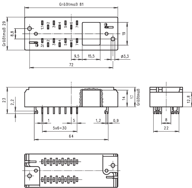
Maßbild Rs 805 202, Blatt 01; 14-polig
