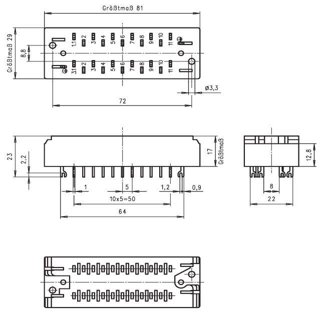
Maßbild Rs 805 202, Blatt 02; 22-polig
