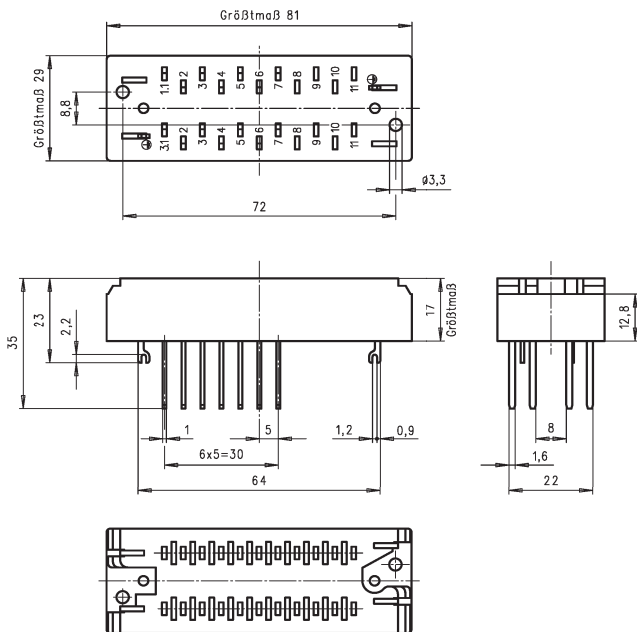
Maßbild Rs 805 255, Blatt 01; 14-polig
