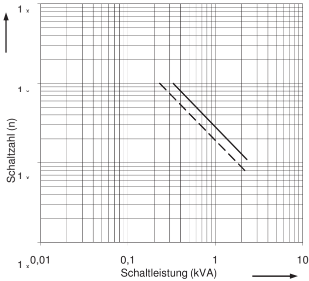
2 RH 01, 2 RH 30 Kontaktwerkstoff AgPd30
