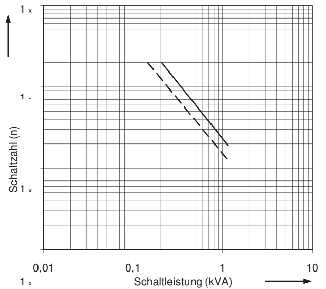
2 RH 02, 2 RH 32 Kontaktwerkstoff AgPd30
