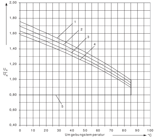
Arbeitsspannungsbereich für folgendes Schaltrelais: 2 RH 01 Normalspannungsbereich (Metallkappe)
