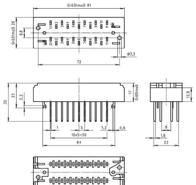
Maßbild Rs 805 255, Blatt 02; 22-polig
