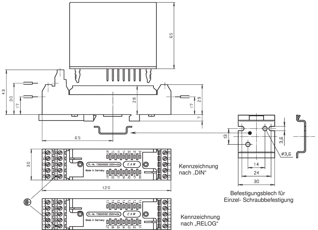
Maßbild Rs 805 042
