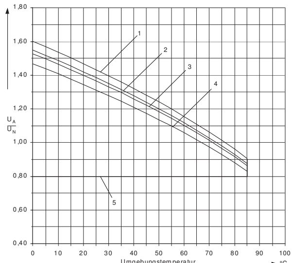
Arbeitsspannungsbereich für folgendes Schaltrelais: 4 RH 10, 4 RH 12 Normalspannungsbereich
