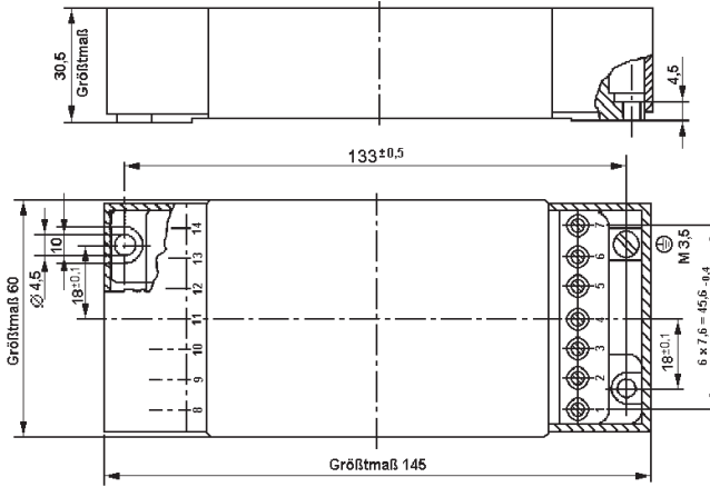
Maßbild Rs 805 541
